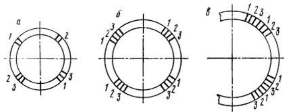
Рис. 3. Схема вырезки образцов для механических испытаний
