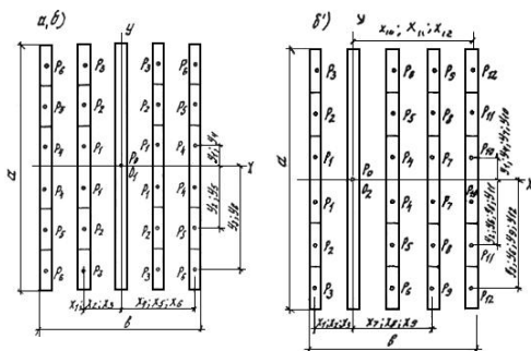
Рисунок Ж.2 - Схемы расположения в плане нагрузок сложного вида, расчетного центра 0, осей координат и разделения следов нагрузок на элементарные площадки
