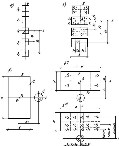
Рисунок Ж.1 - Схемы расположения в плане нагрузок сложного вида, расчетного центра 0, осей координат и разделения следов нагрузок на элементарные площадки
